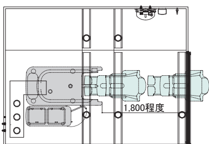
3,000mm×4,000mm (SYK3040C) 参考プラン P72
