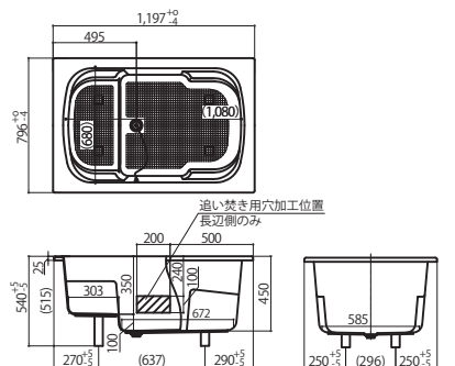
は追い焚き用穴加工(穴芯)範囲を示す
