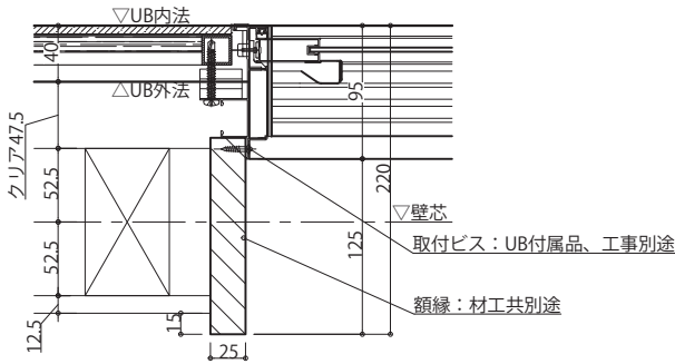
木造 ■ 平面
