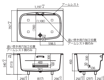
は追い焚き用穴加工(穴芯)範囲を示す
