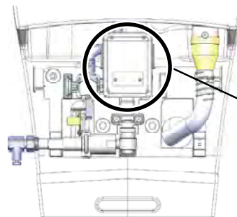
メイン基板は便器の裏側にあります
